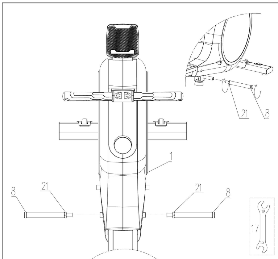
Рисунок 5 — Установка педальных стоек
