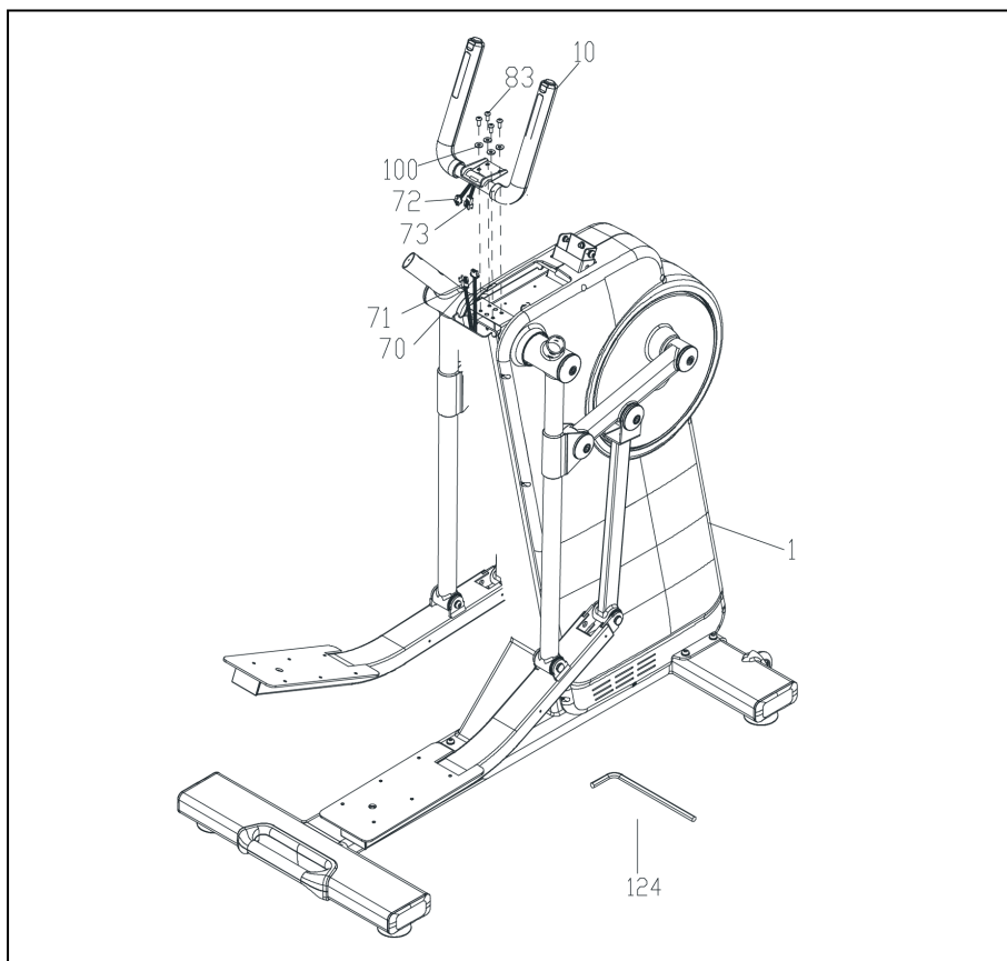
Рисунок 6 — Установка руля
