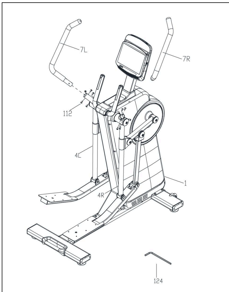
Рисунок 10 — Установка поручней
