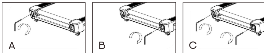
Рисунок 7 – Центровка бегового полотна
